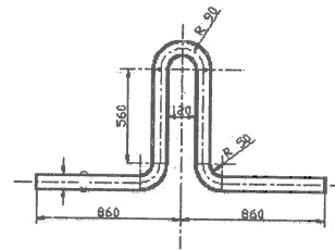
MOORING EYE Ø
